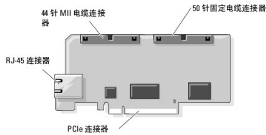
图 1-1. DRAC 5 硬件功能
